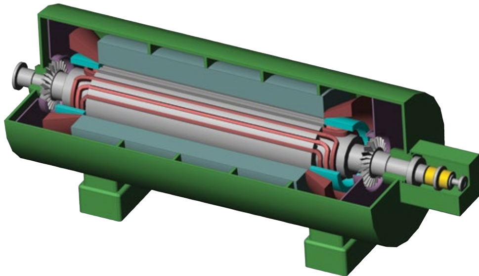
Ensamblajes de colector
